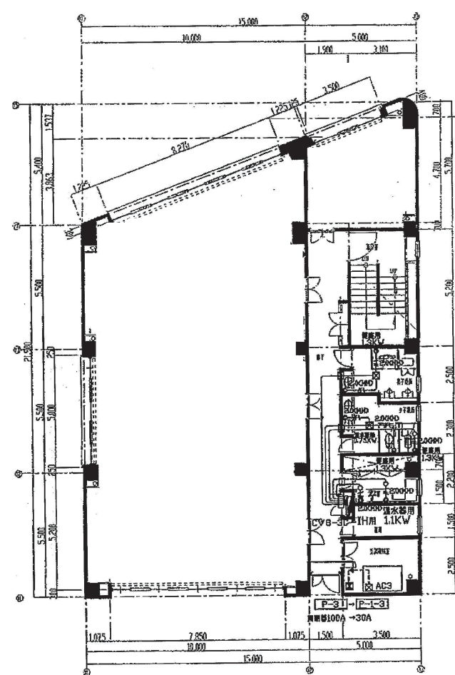
3 F 平面図
