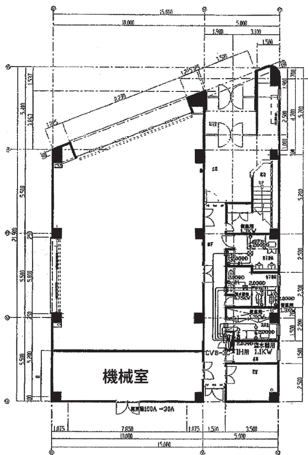
1F平面図
