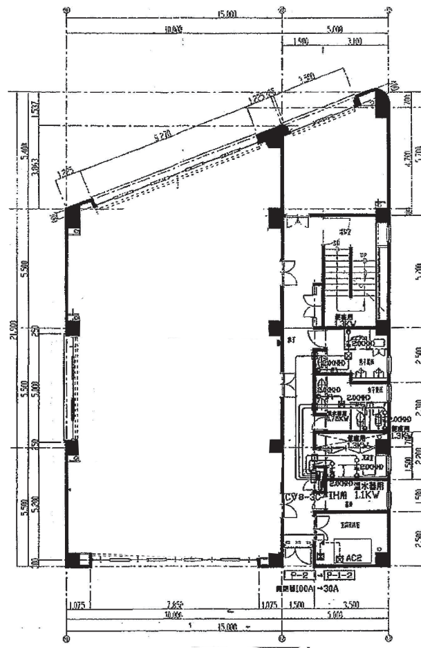
2 F 平面图
